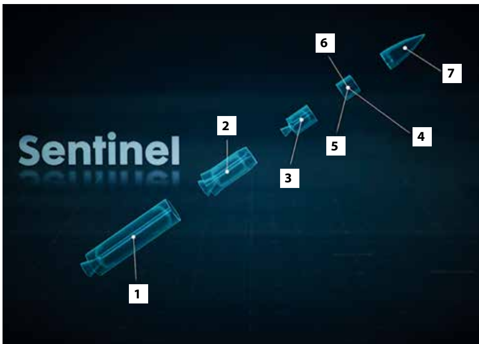
Vývoj mezikontinentální balistické střely LGM-35A Sentinel má na starosti společnost Northrop Grumman, z jejíhož propagačního videa je i tento záběr. Na něm je názorně vidět její konstrukce tvořená třemi motorovými stupni (1, 2 a 3), sekci obsahující inerciální navigační jednotku (4) a aparaturu řídící směr (5) i výšku letu (6) a nakonec bojovou částí (7).
